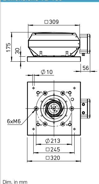
Dimensions VD 180
