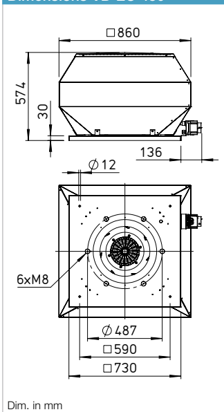
Dimensions VD EC 450
