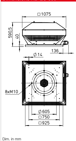
Dimensions RD EC 560
