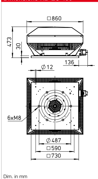
Dimensions RD EC 450
