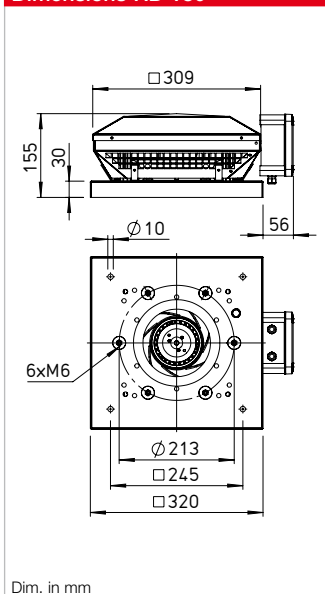
Dimensions RD 180
