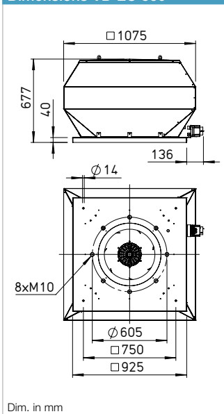
Dimensions VD EC 560
